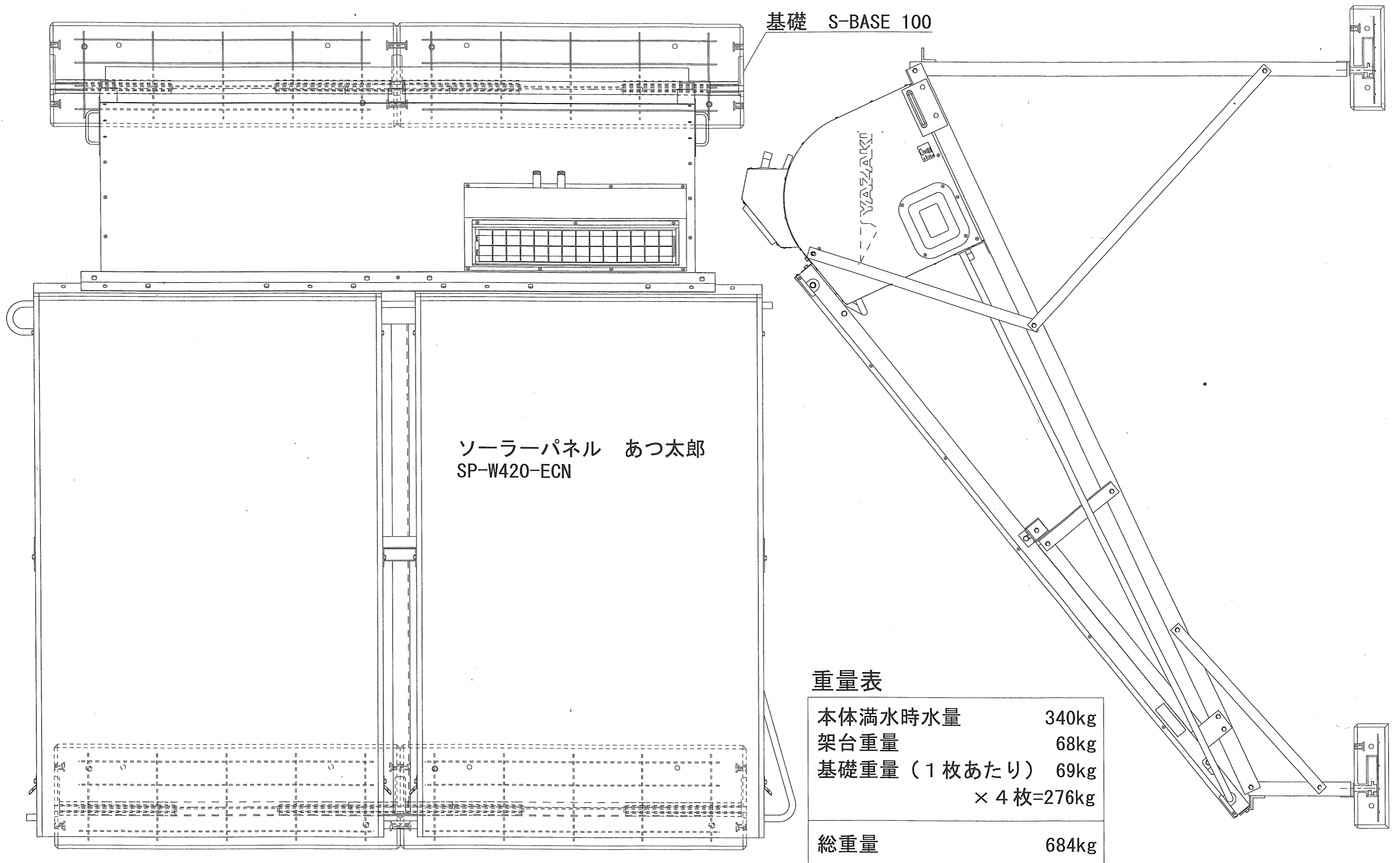
御蔵島 ソーラーパネル設置図
